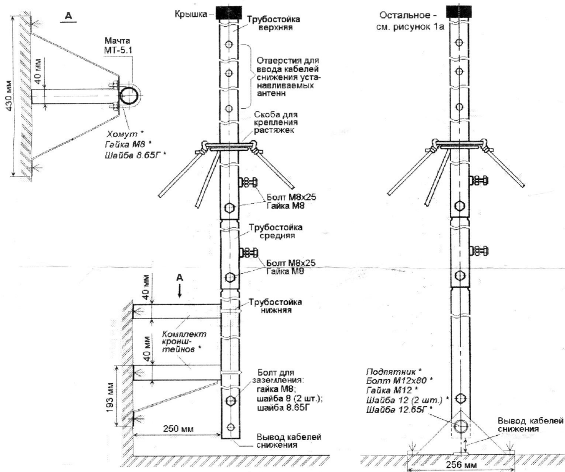
а) с помощью комплекта кронштейнов б) с помощью подпятника Рисунок 1 - Варианты установки мачты
